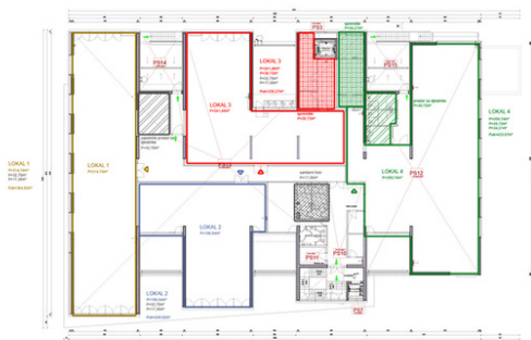
F191 SAMOBOR TLOCRT KATA VARIJANTA 4
