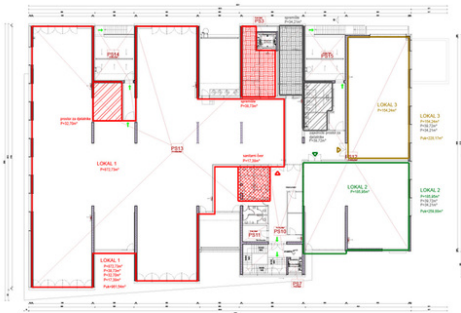
F191 SAMOBOR TLOCRT KATA VARIJANTA 2A
